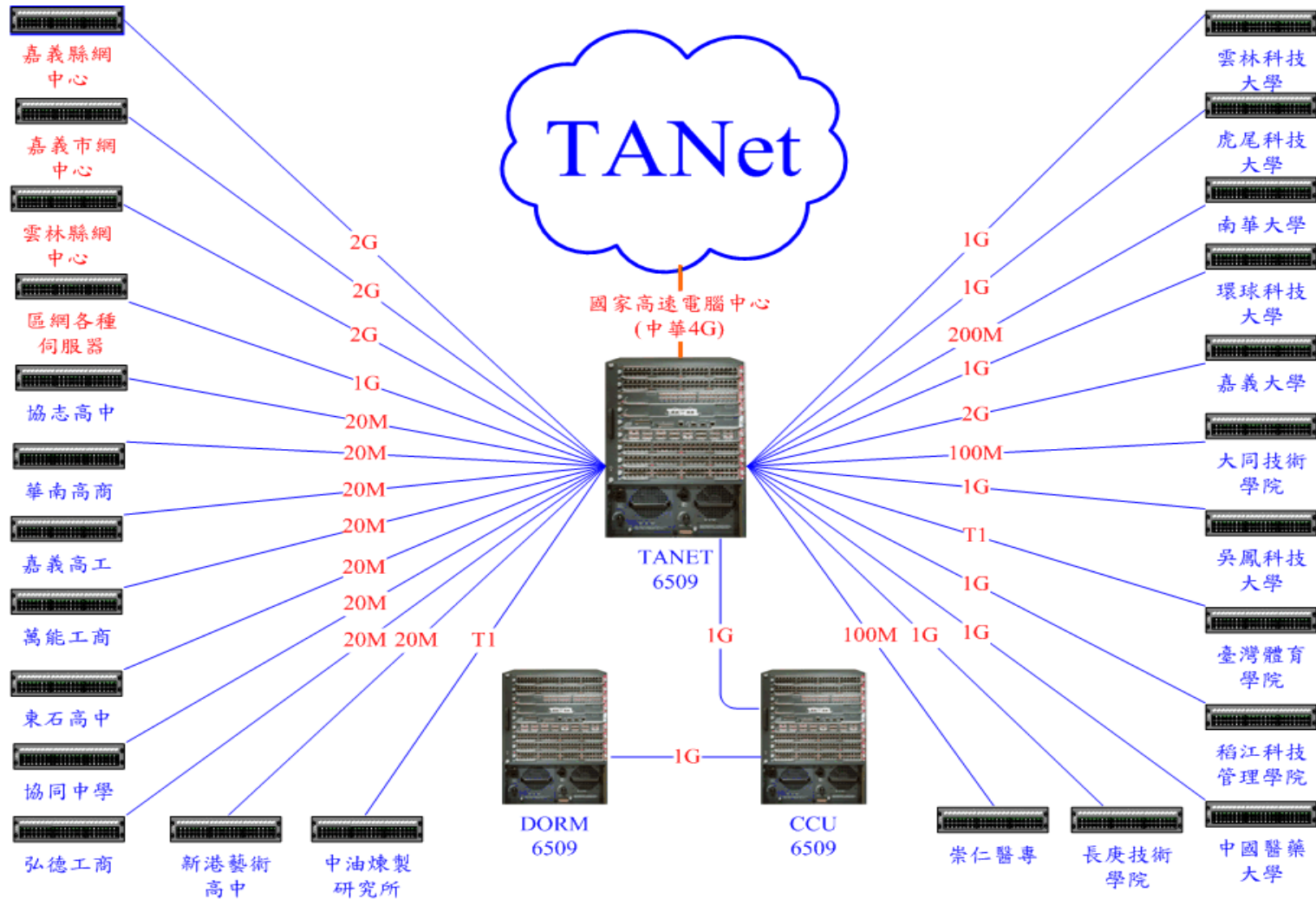
雲嘉區域網路中心各單位連線架構圖
